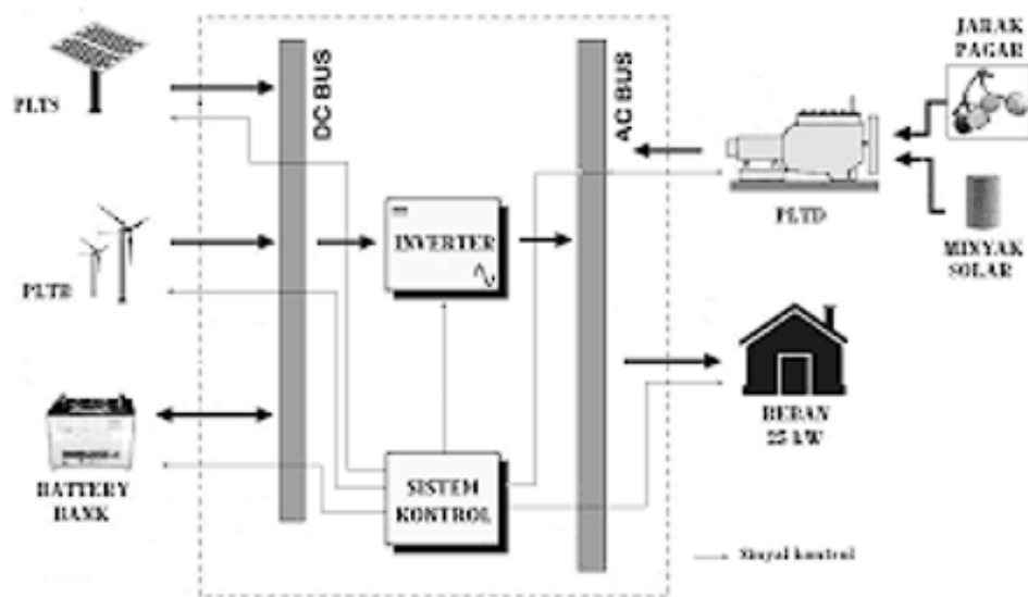
Figure 3. Pembangkit listrik tenaga Hybrid
