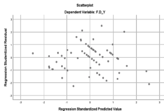
Gambar 1 Uji Heterokedastisitas
