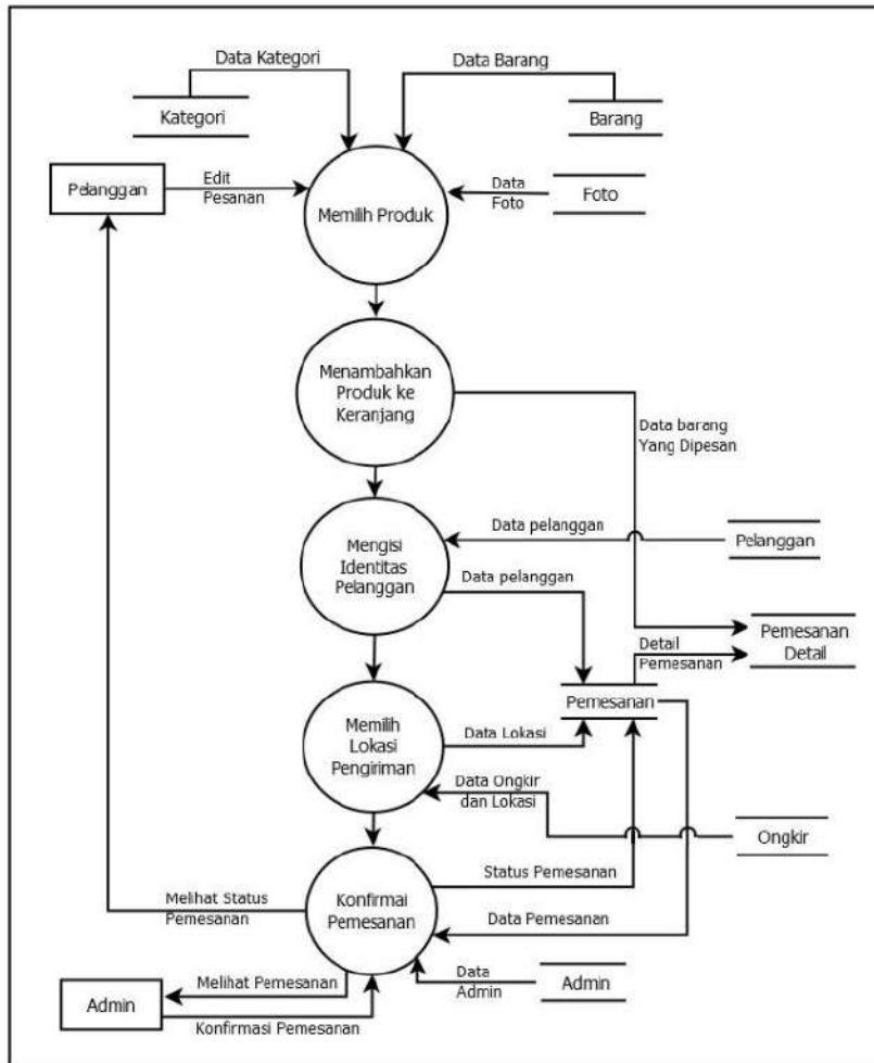
Gambar 2.2 DFD
