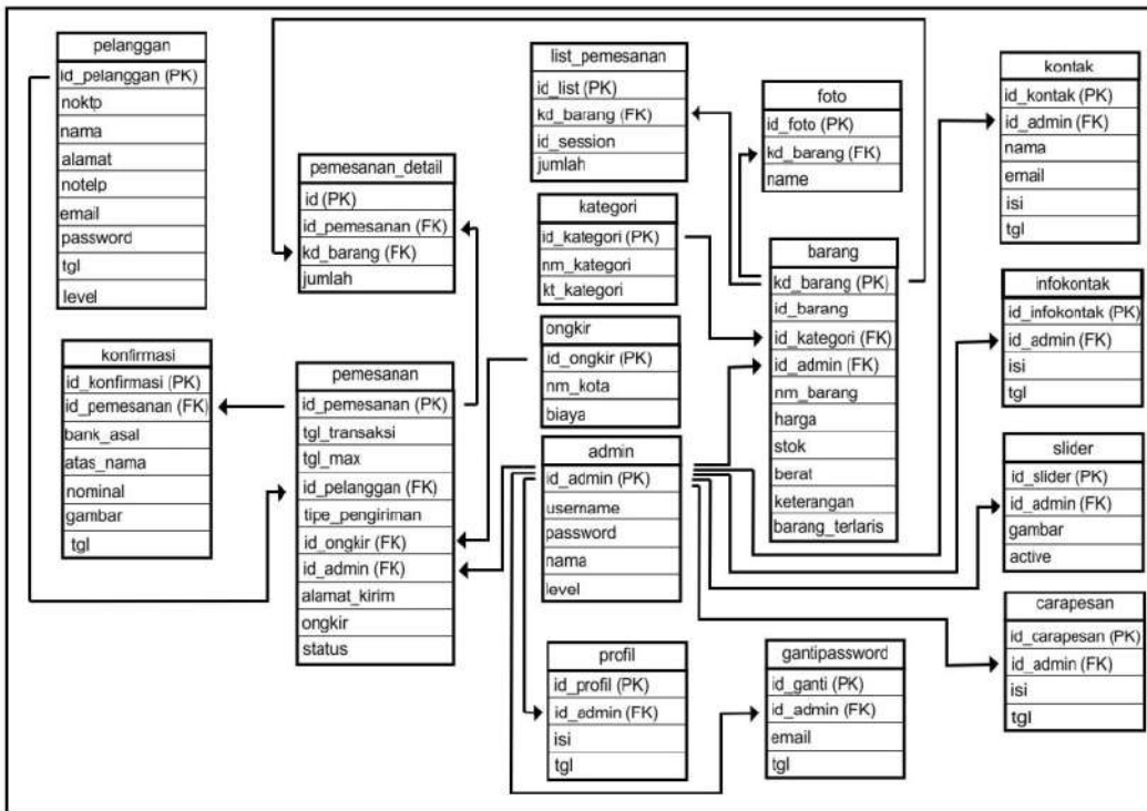
Gambar 2.3 Relasi Tabel
