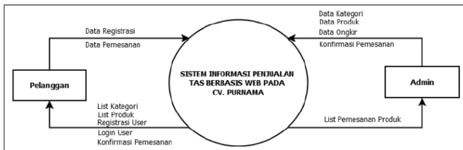
Gambar 2.1 Konteks Diagram
