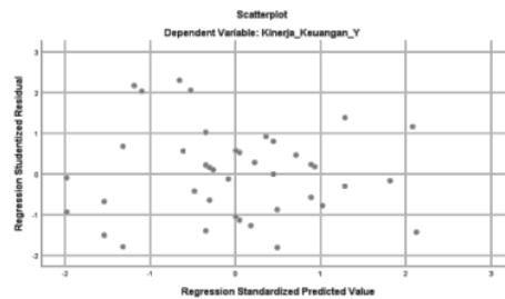
Gambar 1 Uji Heterokedastisitas
