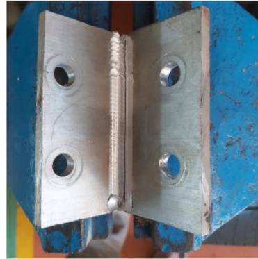
Gambar 4.11 Hasil pengelasan tidak optimal dan terlihat sambungan lepas
