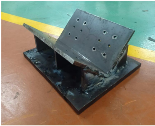
Gambar 2 Jig yang telah jadi
