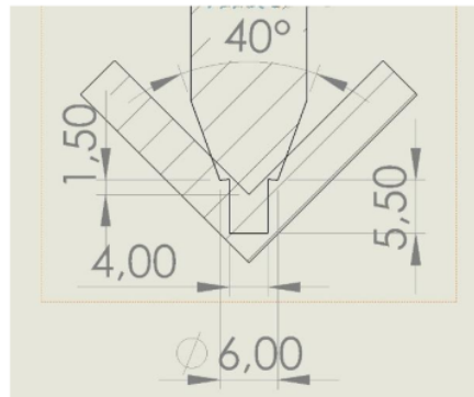
Gambar 3 Dimensi alat pahat yang optimal dalam penelitian
