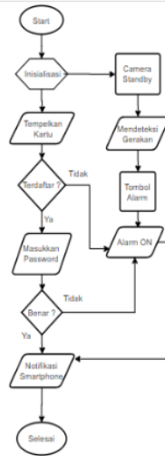
Gambar 12. Flowchart g Brankas Berbasis IoT
