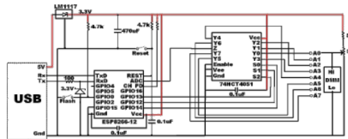
Gambar 10. Esp 8266
