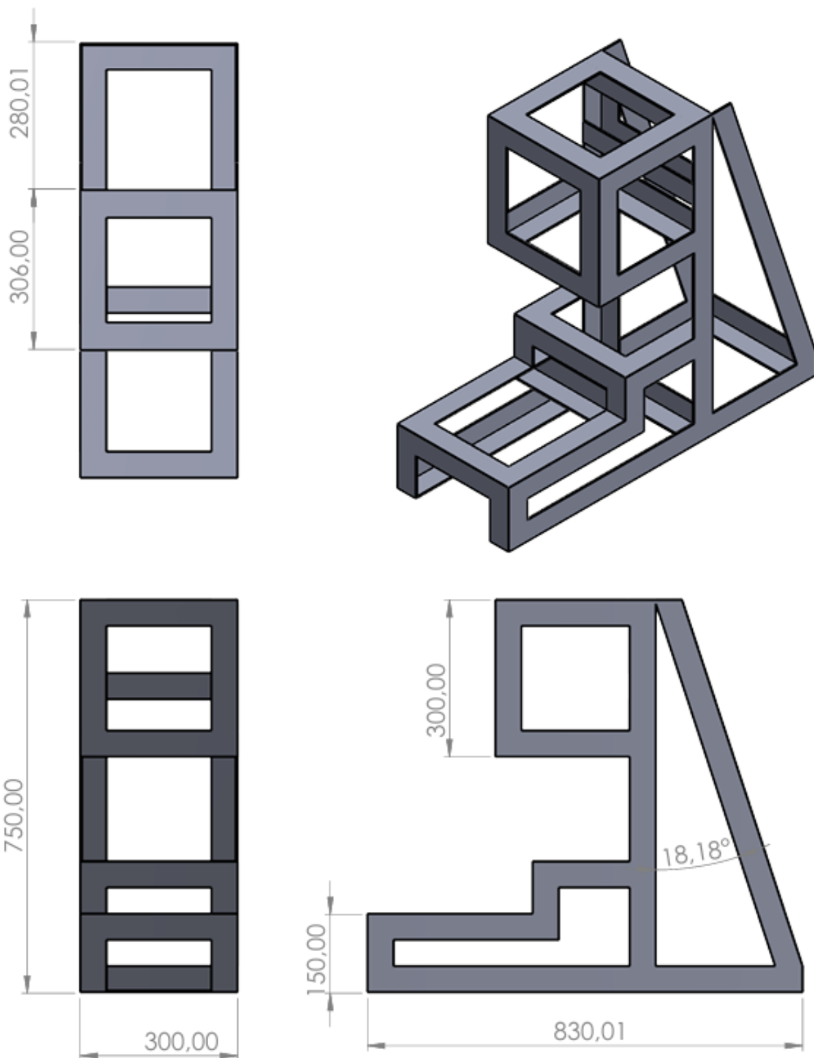
Figure 14. Desain Rangka Alat Pengaduk Adonan Roti
